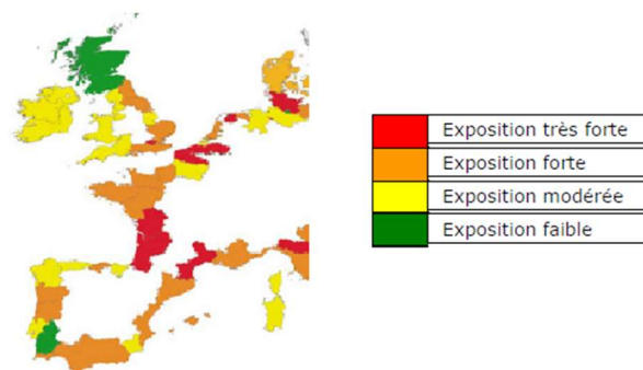
Exposition des côtes européennes à l'érosion côtière
