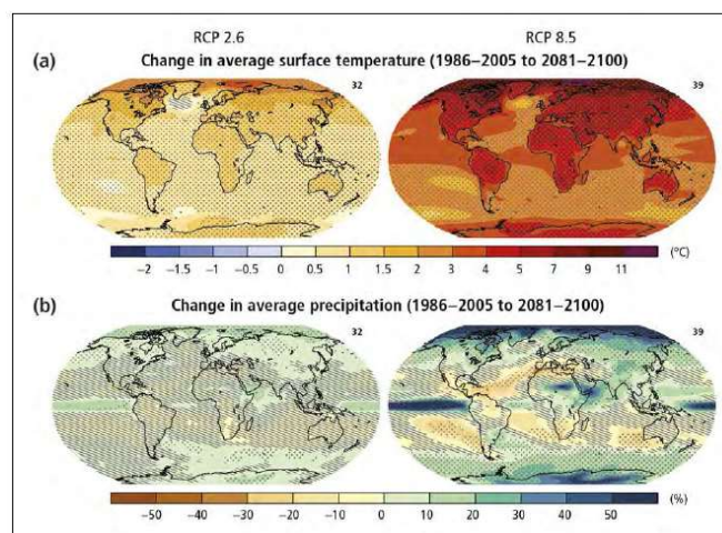
Changement de température moyenne de surface (a) et changement des précipitations moyennes (b) pour 2081-2011 par rapport à 1986-2005 pour les scénarios RCP 2.6 (à gauche) et RCP 8.5 (à droite). (Source : GIEC, Rapport Changements climatiques, 2014)
