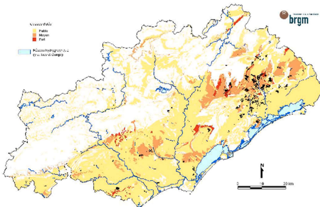
Cartographie de l'aléa retrait gonflement d'argile BRGM - 2005
