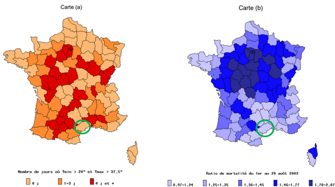
Nombre de jours de très grande chaleur (à gauche) et ratio de mortalité (à droite) pour la période du 01 au 21 août 2003 (Source : INSERM, 2004)
