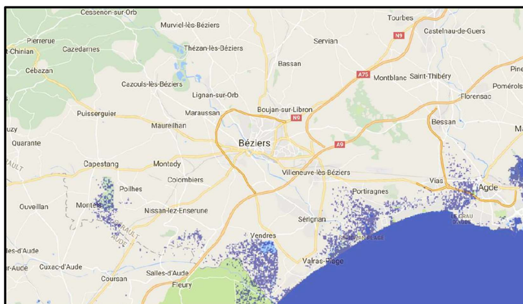
Simulation de l'impact d'une montée du niveau des eaux marines (1m) sur la zone littorale de La Domitienne
